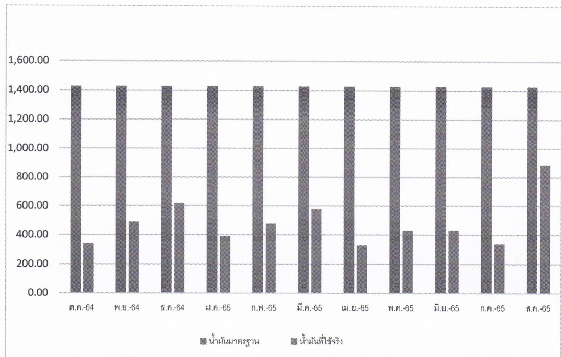
แผนภูมิ ๒ สถิติการใช้พลังงานเชื้อเพลิง เปรียบเทียบกับค่ามาตรฐานการใช้พลังงาน
